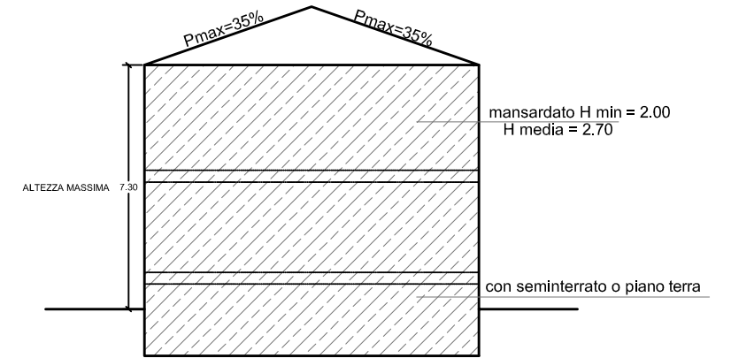
SEZIONE 1-1
