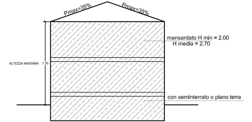
SEZIONE 1-1
