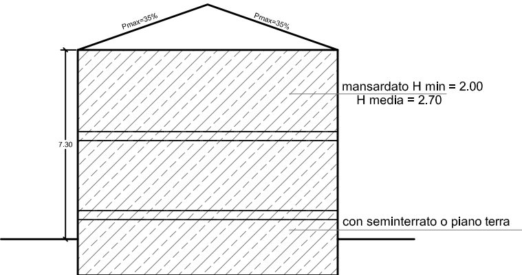
SEZIONE 1-1
